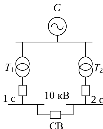
Рисунок 2. Схема к практической работе «Проверка сечения шин на термическую стойкость к токам короткого замыкания»
